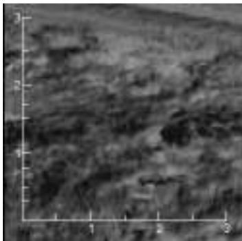
Рисунок 22 – Измерительная шкала
