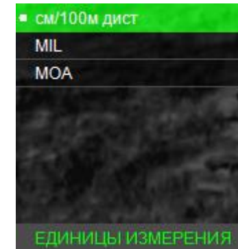
Рисунок 20 – Единицы измерения
