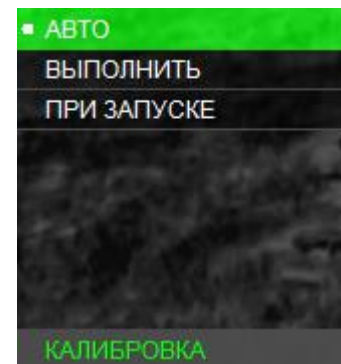
Рисунок 27 – Калибровка
