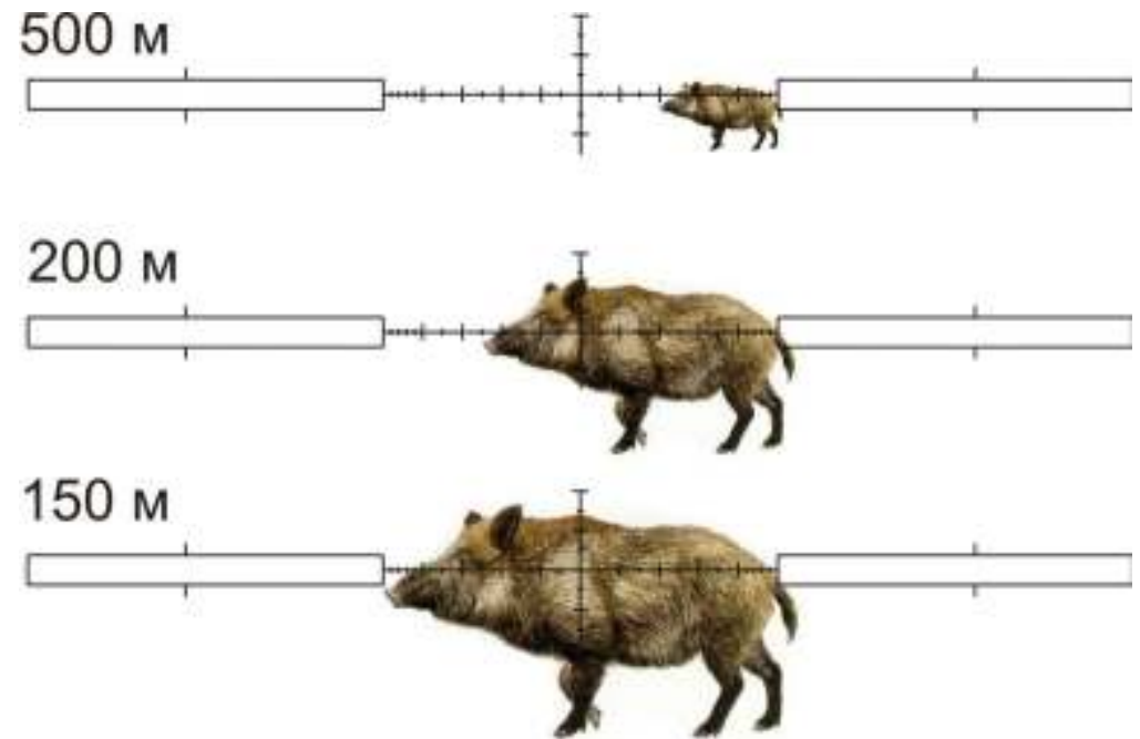
Рисунок 33 – Определение расстояния до цели по сетке «Mil-Dot»
