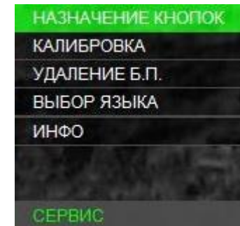
Рисунок 25 – Сервис
