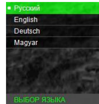
Рисунок 28 – Выбор языка
