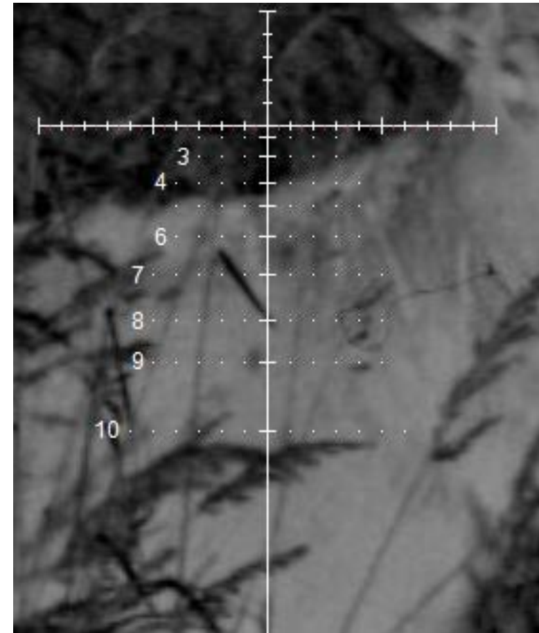
Рисунок 17 – Сетка «БАЛЛИСТИЧЕСКАЯ-2»
