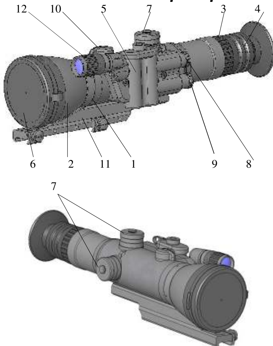
Рис. 1 Прибор «Dedal-445-A»
